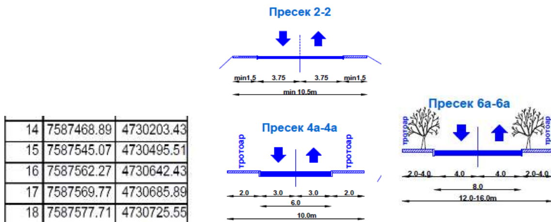
Регулација и нивелација из ППР са изменама и допунама
